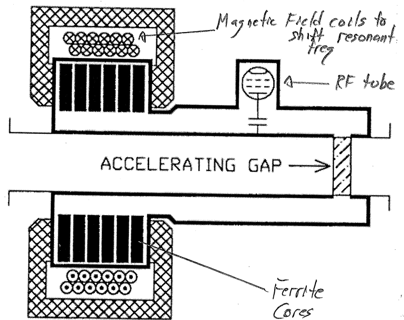
Fig. 20 Los Alamos / TRIUMF cavity
